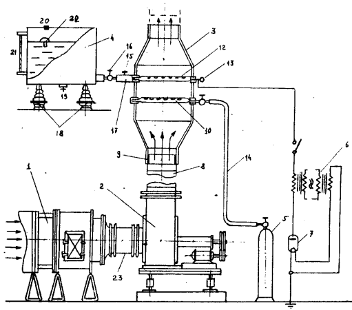
Рис. 5. Водяной высоковольтный аэроионизатор и кислородная система кондиционера: 1 – секция кондиционера; 2 – вентиляционная установка; 3 – корпус аэроионизатора; 4 – водяной бак; 5 – кислородный баллон; 6 – трансформатор; 7 – кенотрон; 8 – диффузор (патрубок из просмоленного брезента); 9 – нижний переходной направляющий патрубок (из жести); 10 – стеклянная трубка с отверстиями для подачи кислорода; 11 – верхний переходной направляющий патрубок (из жести); 12 – стеклянная трубка с отверстиями для подачи воды; 13 – электрод высокого напряжения; 14 – шланг для кислорода; 15 – пробный кран; 16 – регулирующий вентиль; 17 – водяная магистраль (для подвода воды к стеклянной трубке); 18 – высоковольтные изоляторы; 19 – спусковой кран; 20 – наливной патрубок; 21 – водомерное стекло; 22 – поплавковый клапан; 23 – конфузор (соединительный патрубок последней секции кондиционера с вентиляционной установкой).
